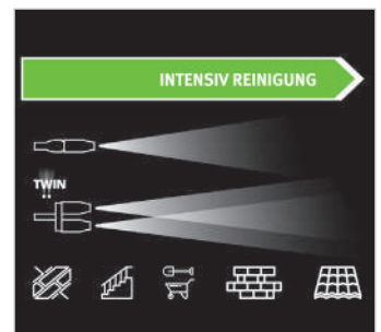
Stufe 2: Modus mit 2 Pumpen , dadurch höherer Arbeitsdruck und Wasserfluss für starke Verschmutzungen
